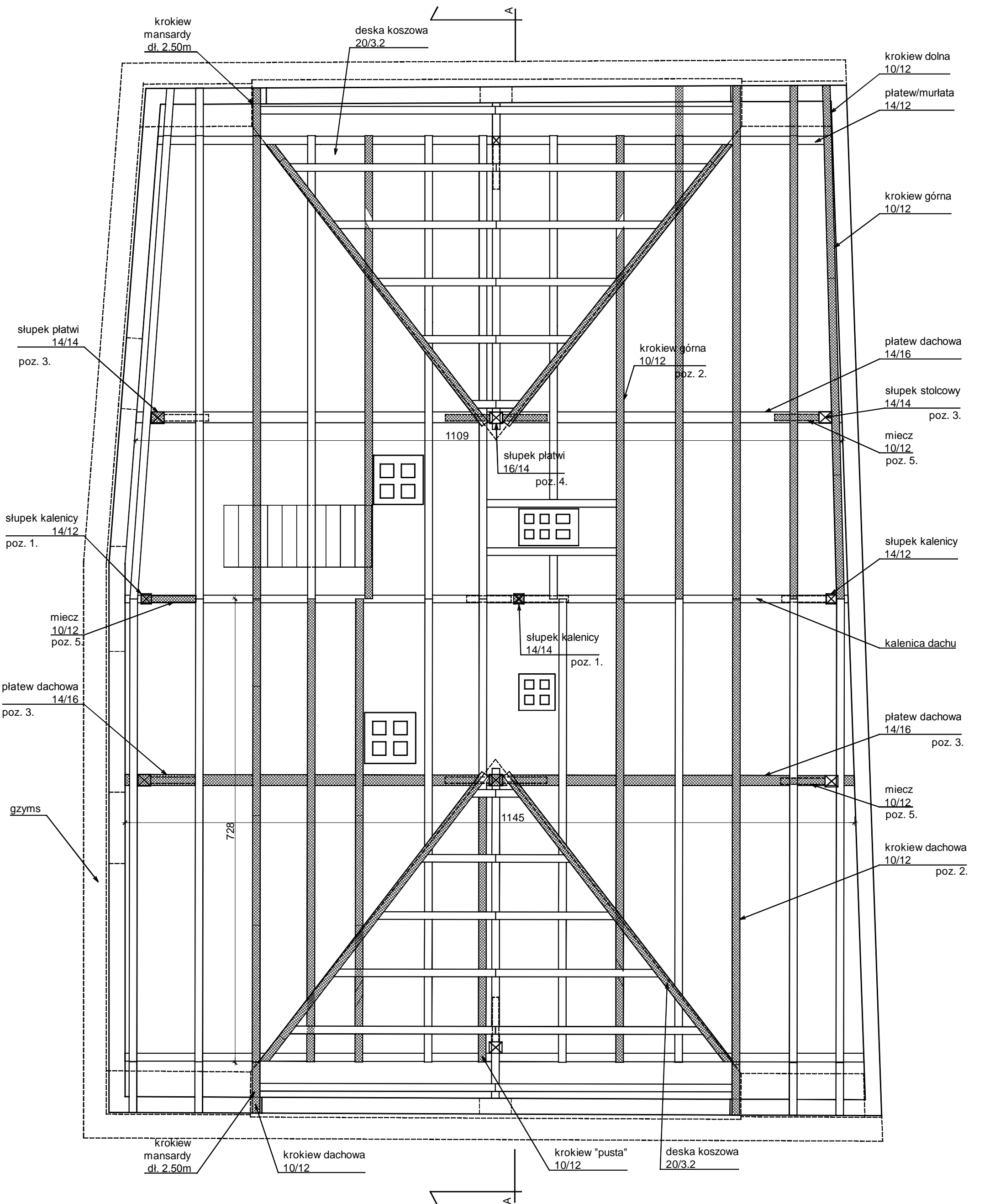
rzut więźby - elementy do wymiany
